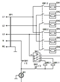
Рис.1.1 Схема электрическая на ТПП-18
