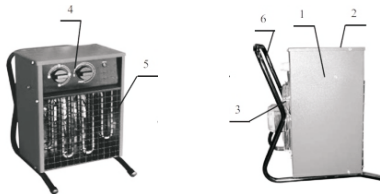
Рис. 1 Тепловентилятор
