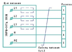
Рис. 3 Схема подключения розетки к стационарной сети
