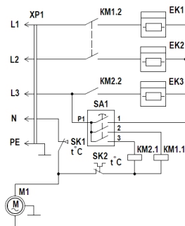
Рис.1.1 Схема электрическая на ТПП-12, ТПП-15 Вилка
